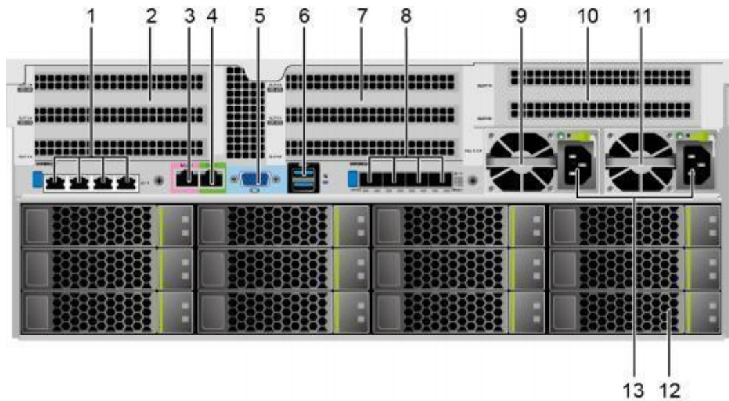
图 4.2：后面板组件
