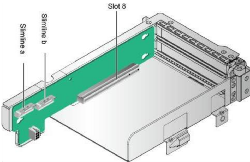
图 4.13: 1x16 Riser 卡 7
