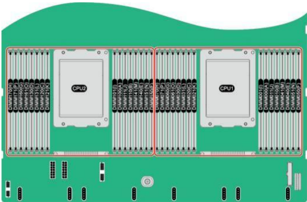
图 6.1: DIMM 安装位置 (鲲鹏 920 7260、5250处理器)
